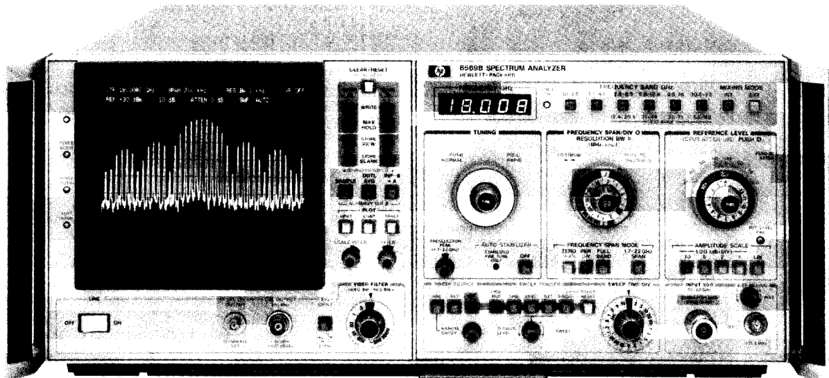
HP 8569B
